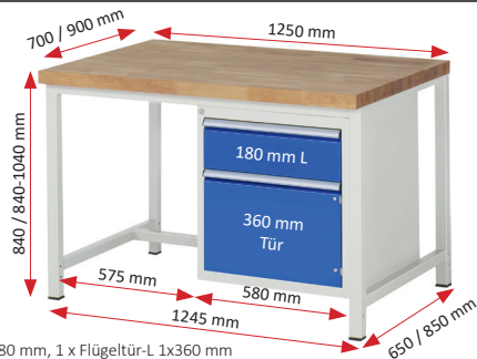
1 x Schublade-L 1x180 mm, 1 x Flügeltür-L 1x360 mm
